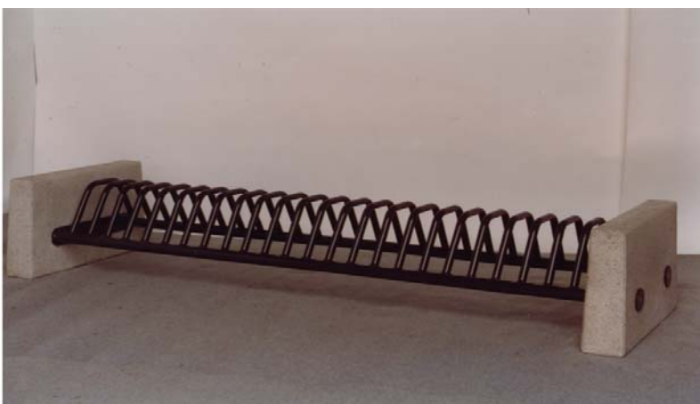
Portabici arredo urbano art. 12305 5 posti dim. 2240 x 700 h 420 mm kg = 27 art. 12307 7 posti dim. 2790 x 700 h 420 mm kg = 33 art. 12309 9 posti dim. 3240 x 700 h 420 mm kg = 41
